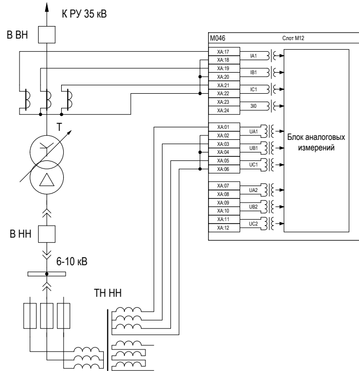
Рисунок Г.1 – Подключение аналоговых цепей трансформаторов тока и напряжения двухобмоточного трансформатора 35 кВ к устройству
